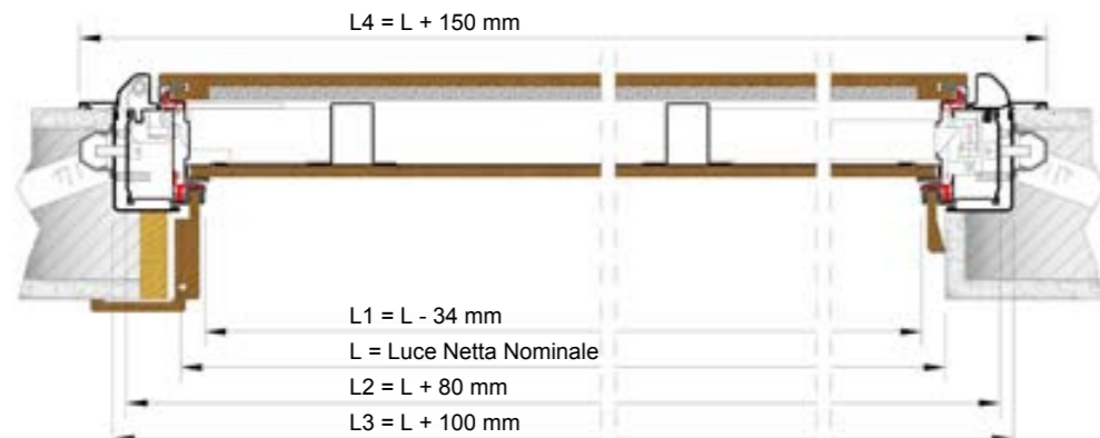
Sezione Orizzontale
